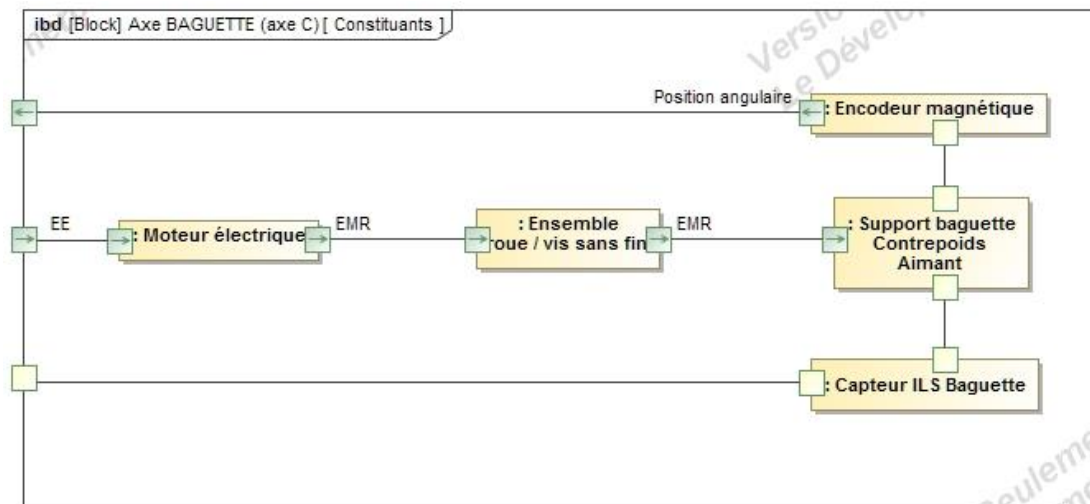
Diagramme de bloc interne (SysML Internal Block Diagram)
