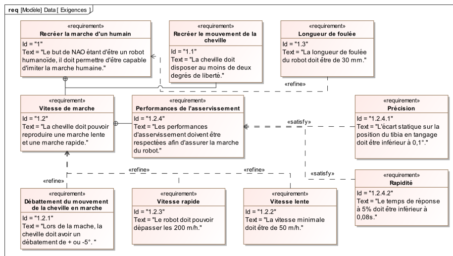
Figure 2: Diagramme des exigences
